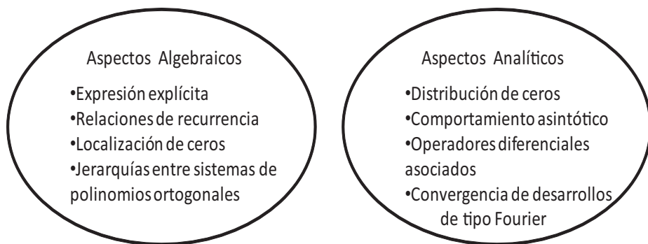
Figura 1: Aspectos algebraicos y analíticos presentes en la TPO.
