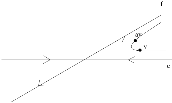
Figura 3.7: Si hay ángulos pequeños, hay puntos cuya imagen está cerca.
