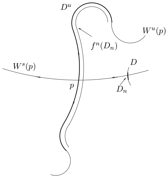
Figura 2.5: Lema de Incliniación
